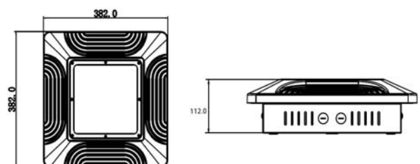
WSLI-CP100/-CP150 (ceiling)
